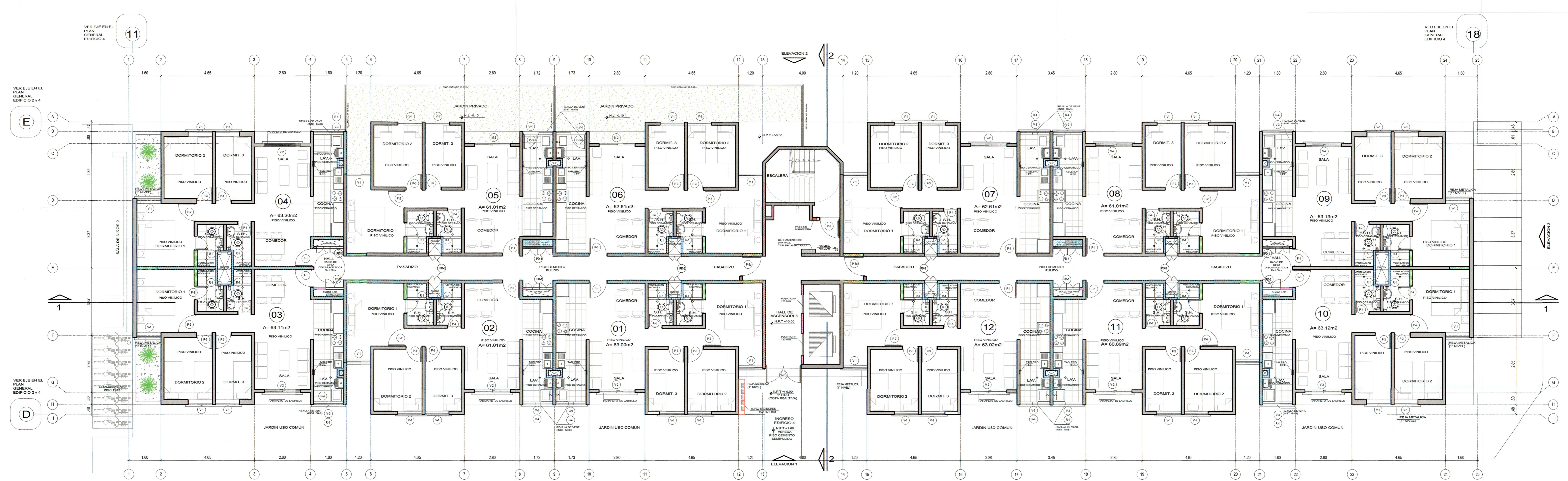
PLANTA 1º PISO - EDIFICIO 4 ESC.: 1/75
