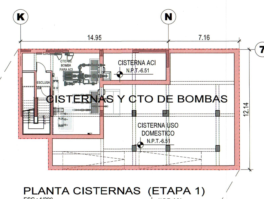
PLANTA CISTERNAS (ETAPA 1) ESC. 1:500
