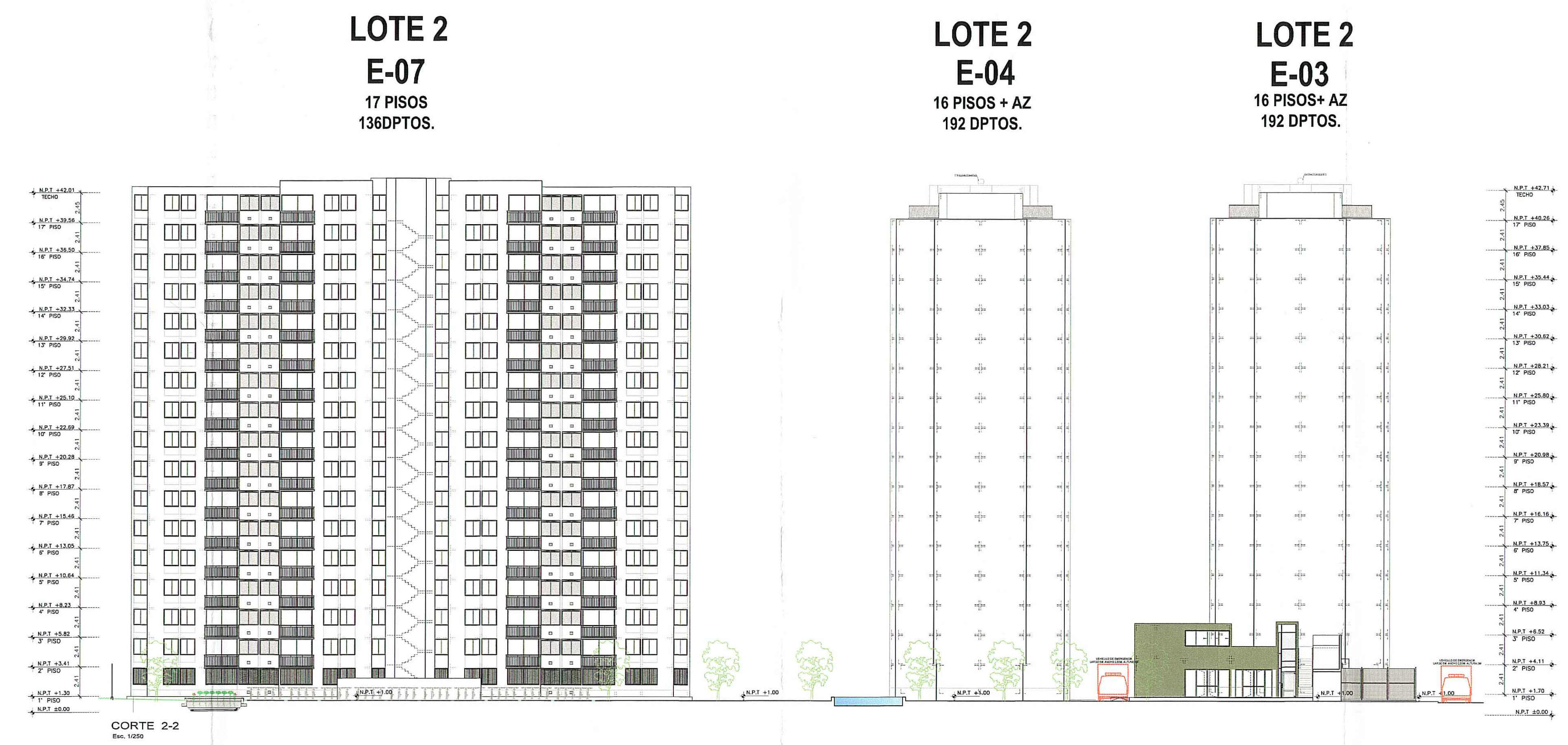
CORTE 2-2 Esc. 1/200
