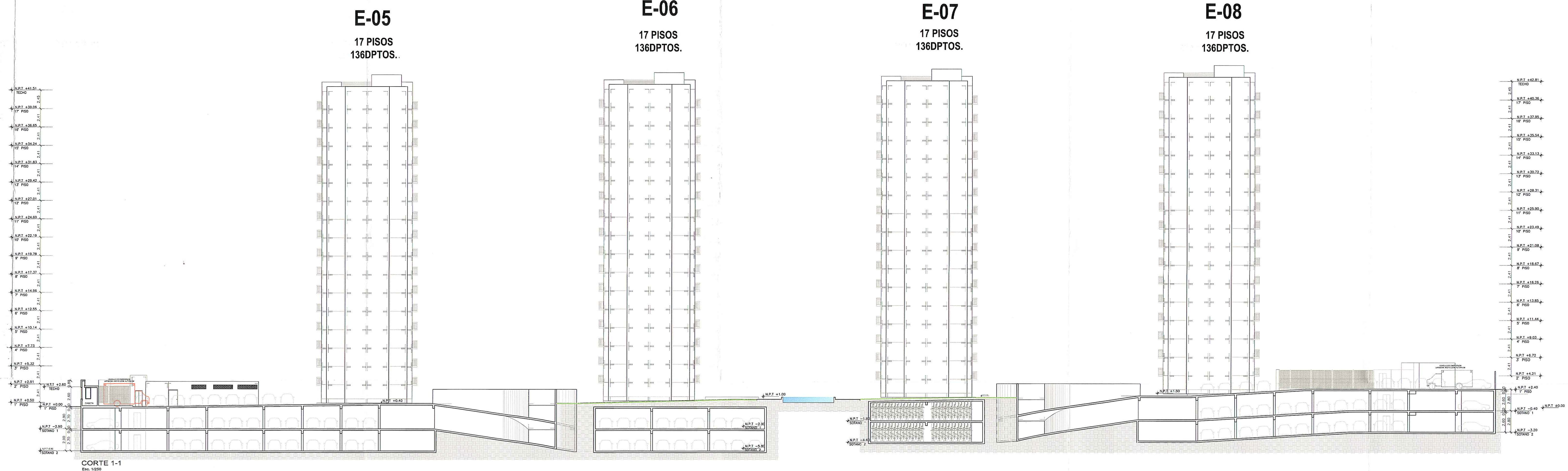
CORTE 1-1 Esc. 1/200
