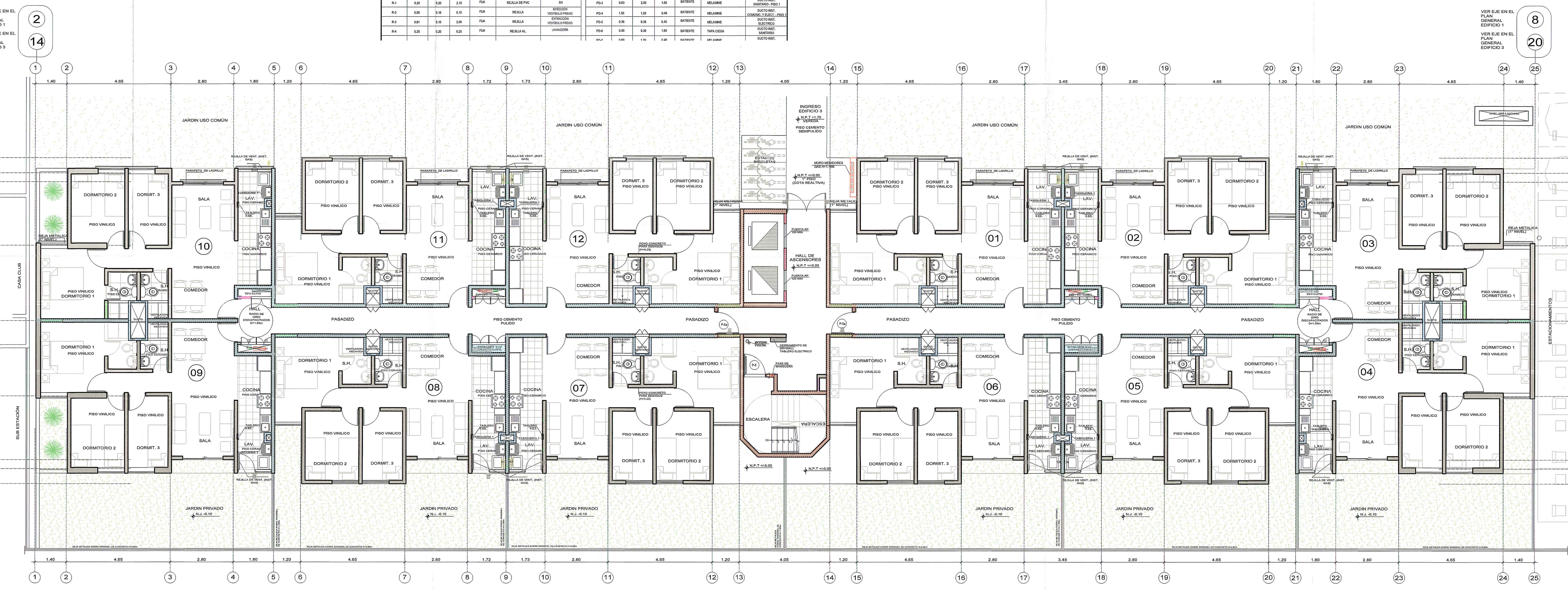
PLANTA 1º PISO - EDIFICIO 3 ESC.: 1/75
