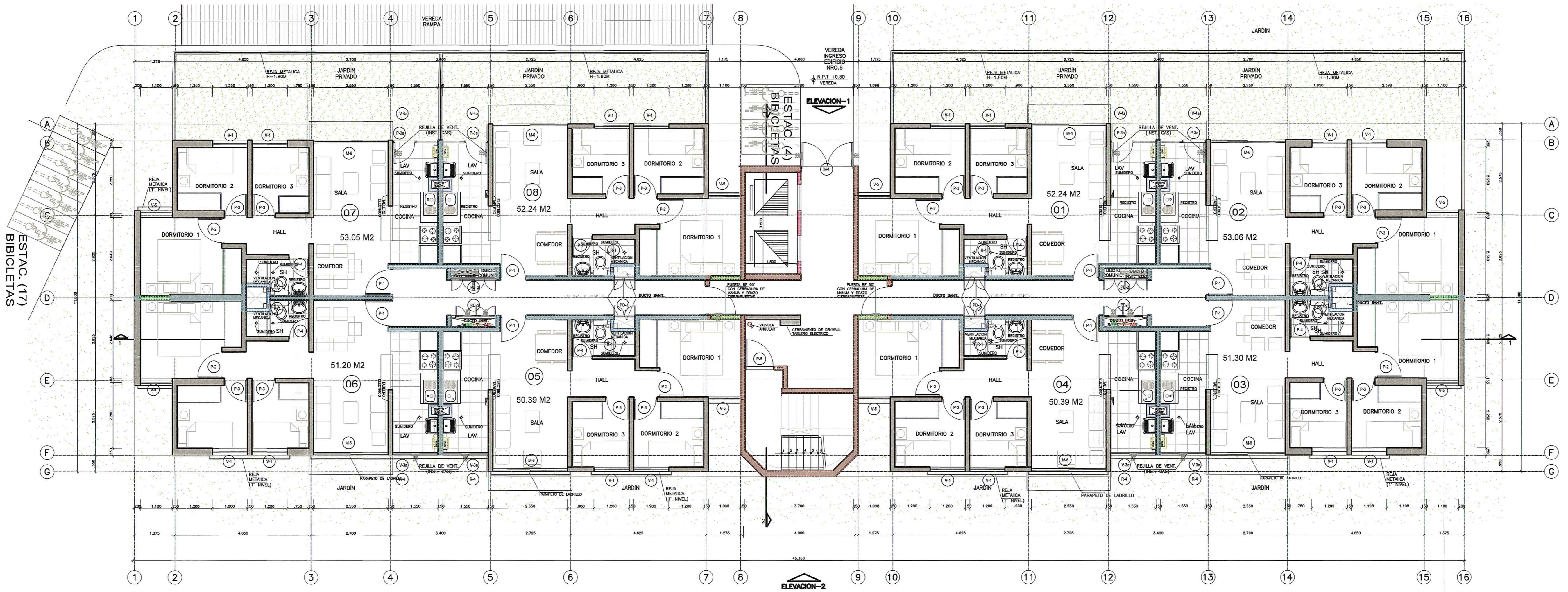
PLANTA 1º PISO - EDIFICIO 6 ESQ.- 1775
