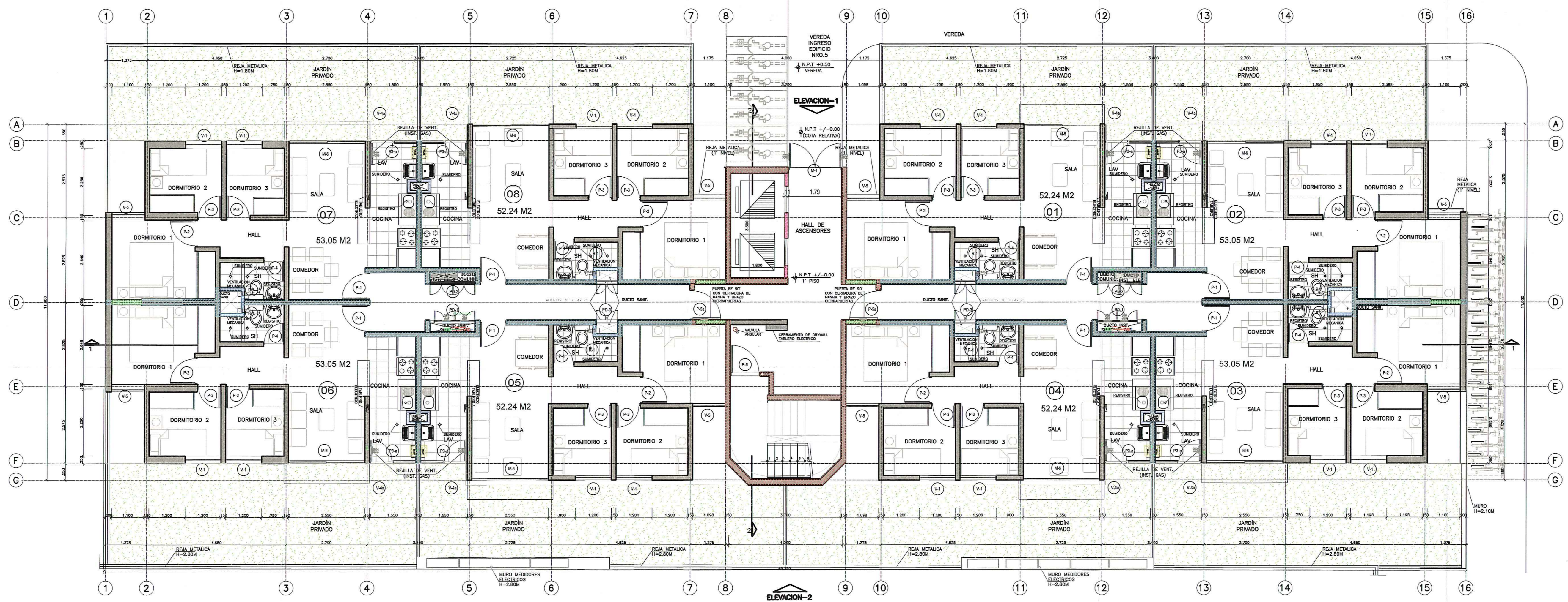
PLANTA 1º PISO - EDIFICIO 5 ESQ.- 1775
