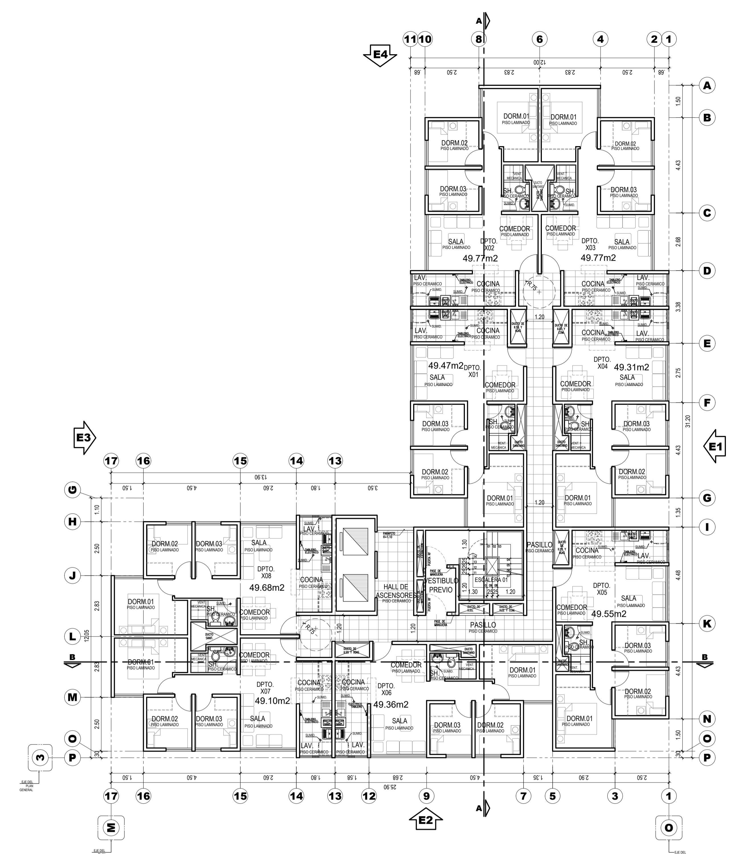
PLANTA TÍPICA PISOS 2 AL 21 ESCALA: 1/100
