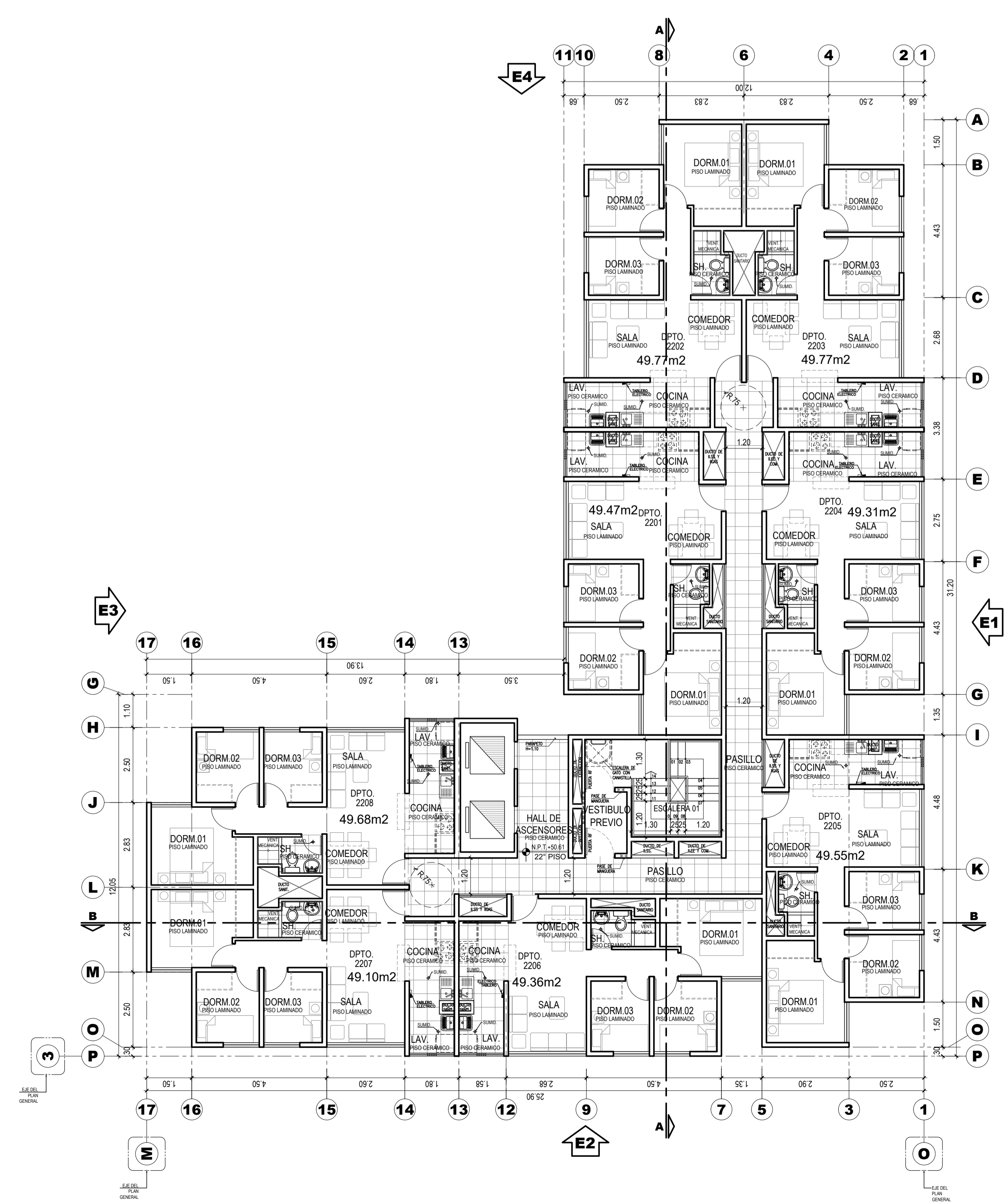
PLANTA PISO 22 ESCALA: 1/100
