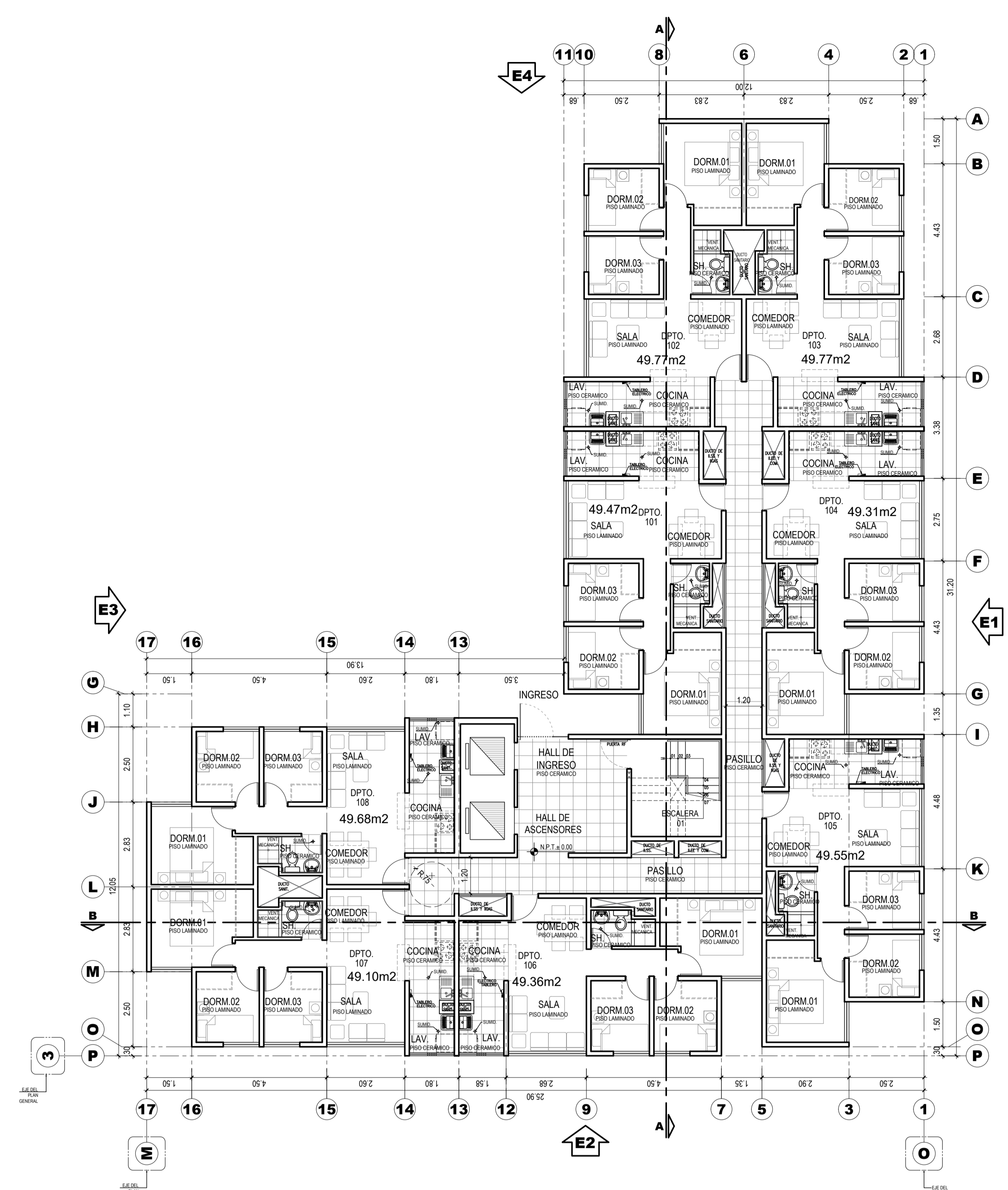
PLANTA PISO 1 ESCALA: 1/100
