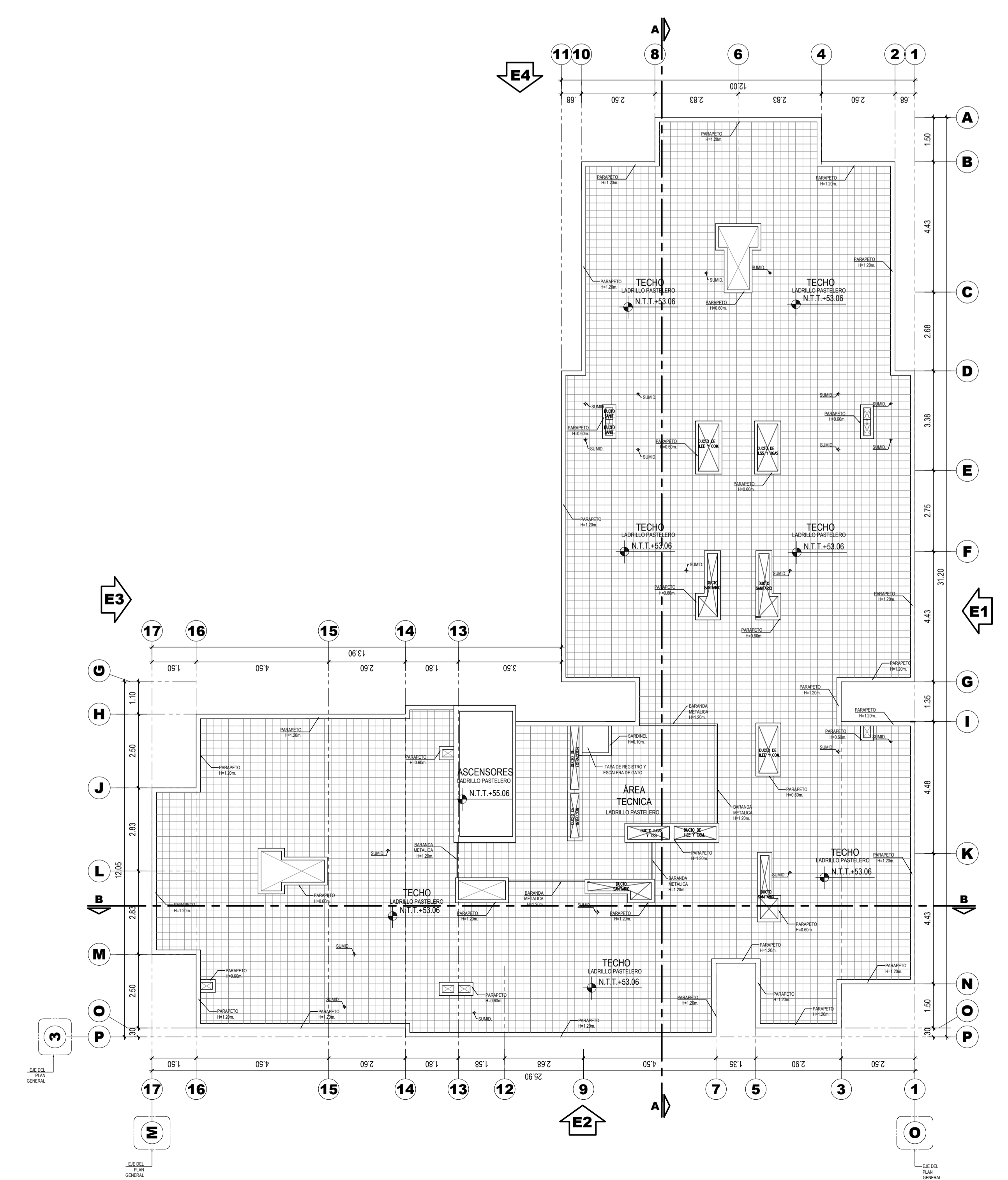
PLANTA TECHO ESCALA: 1/100
