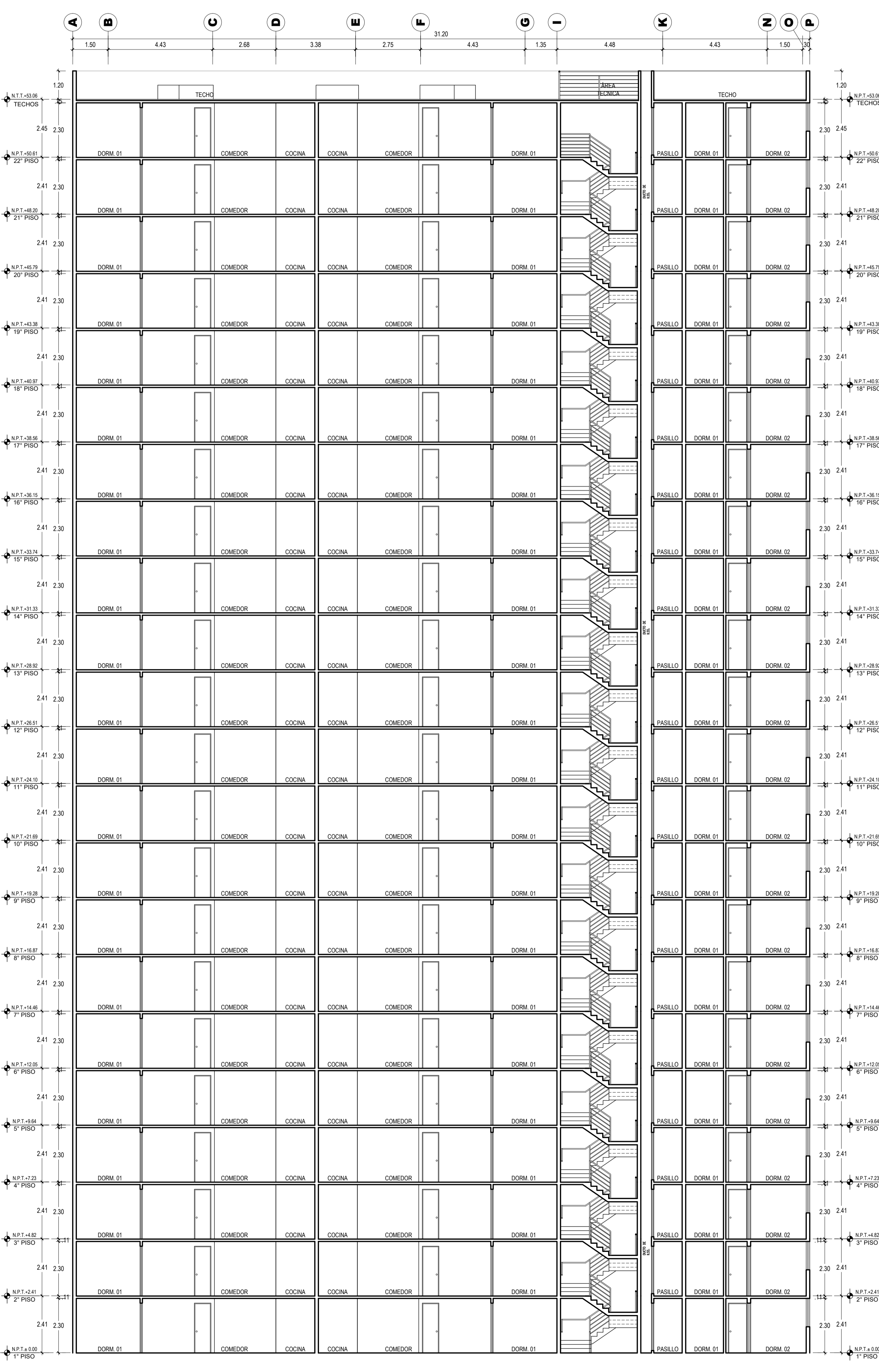
CORTE A ESCALA: 1/100
