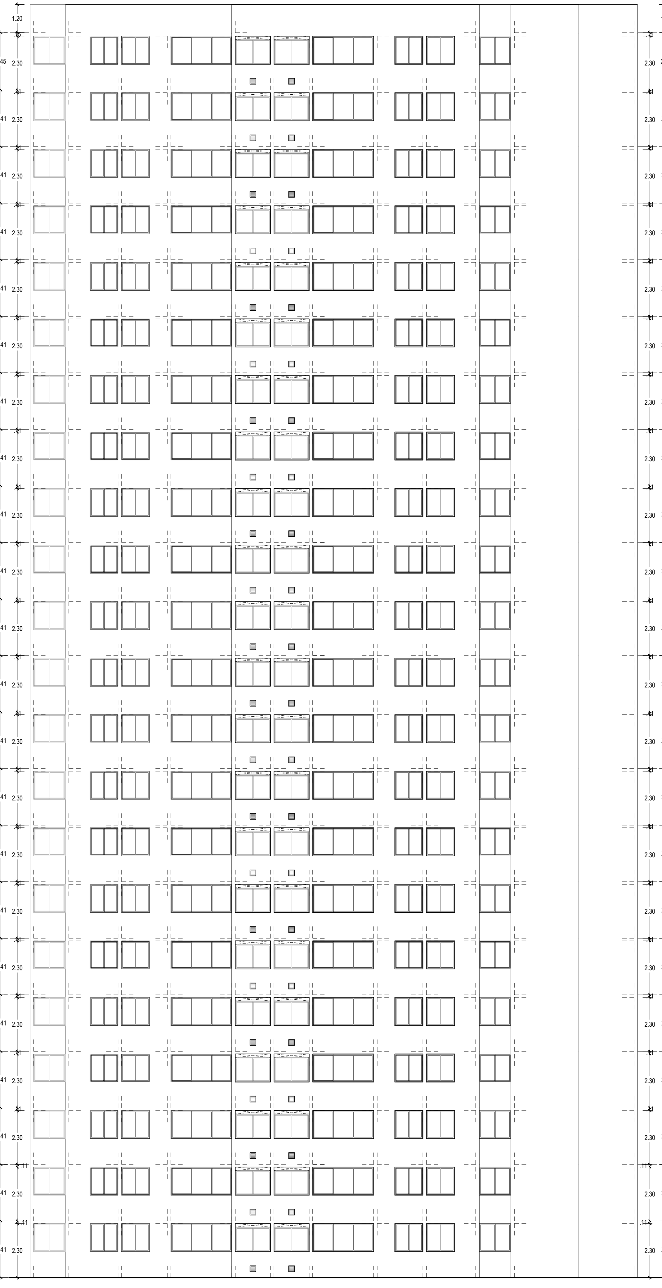
ELEVACION 2 ESCALA 1/50
