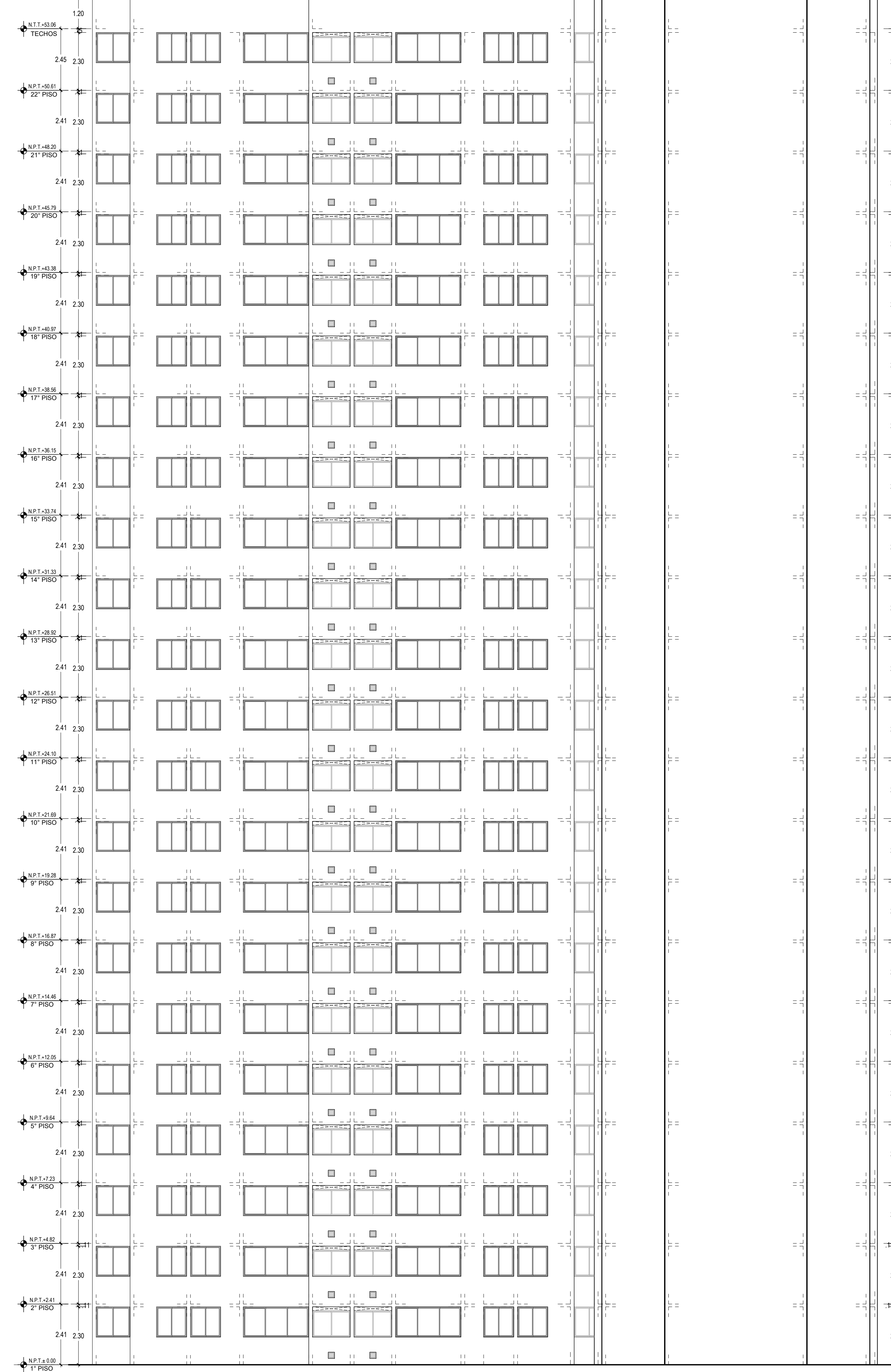
ELEVACION 3 ESCALA 1/50
