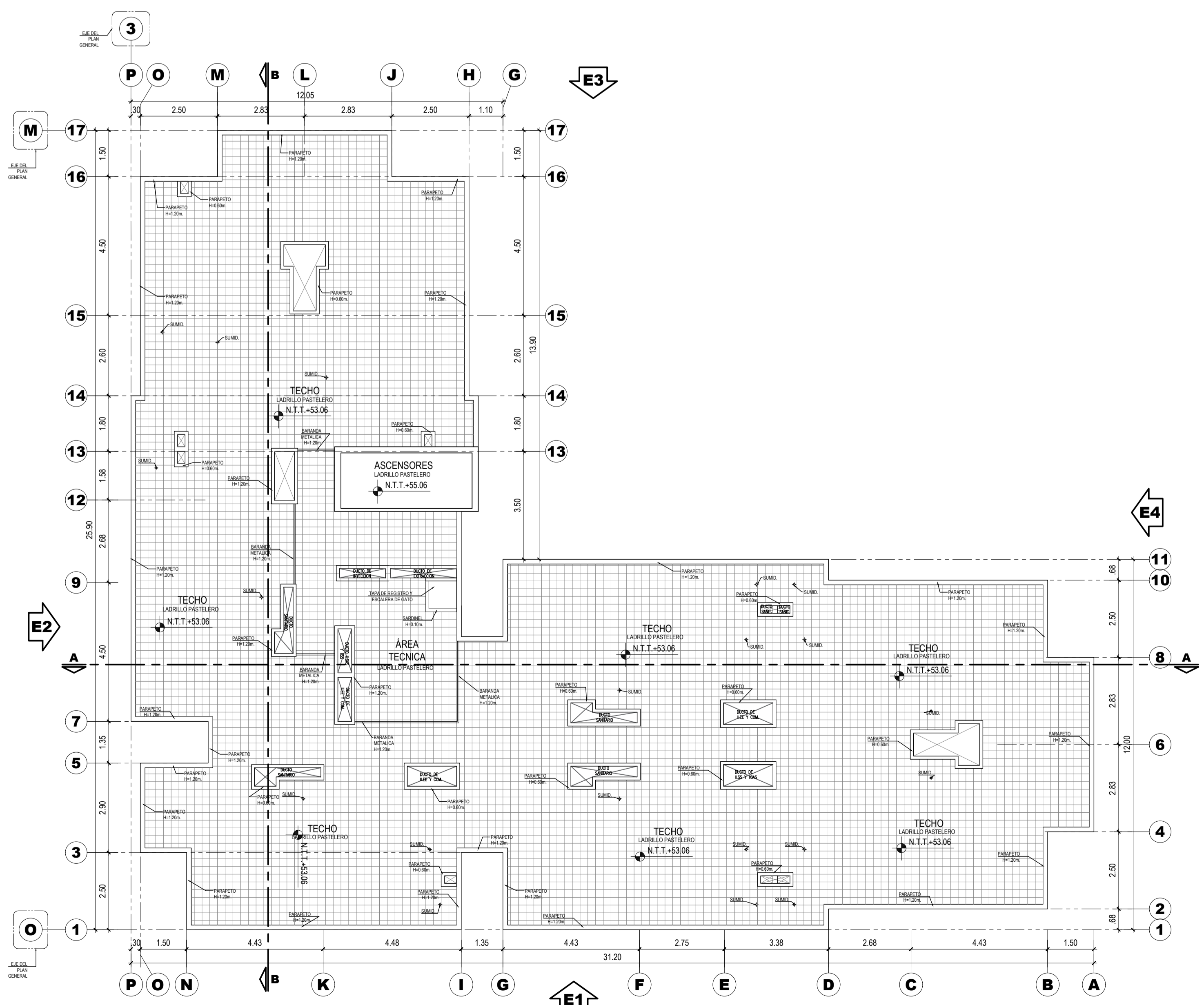
PLANTA TECHO ESCALA: 1/100
