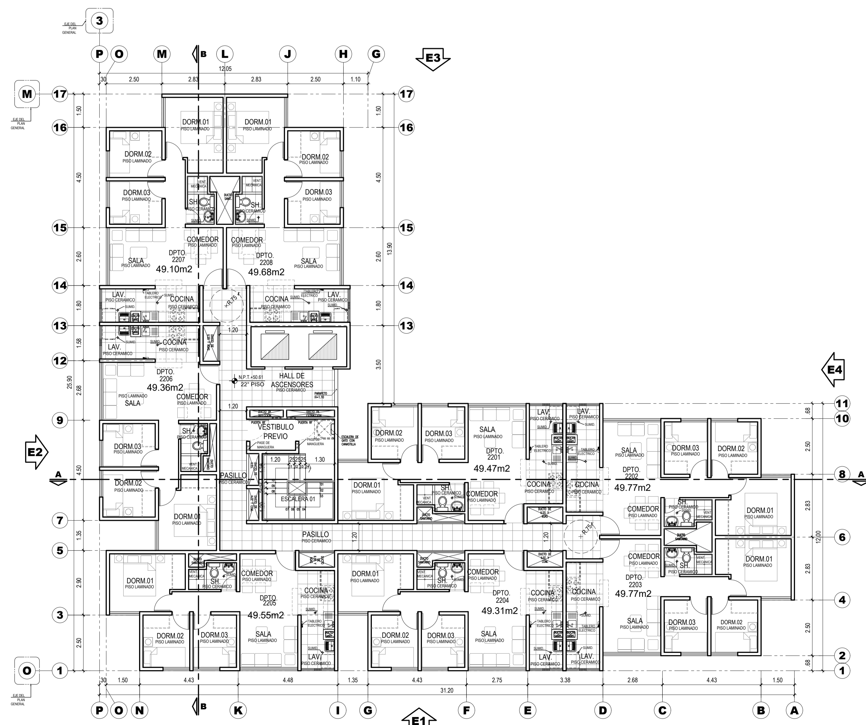
PLANTA PISO 22 ESCALA: 1/100
