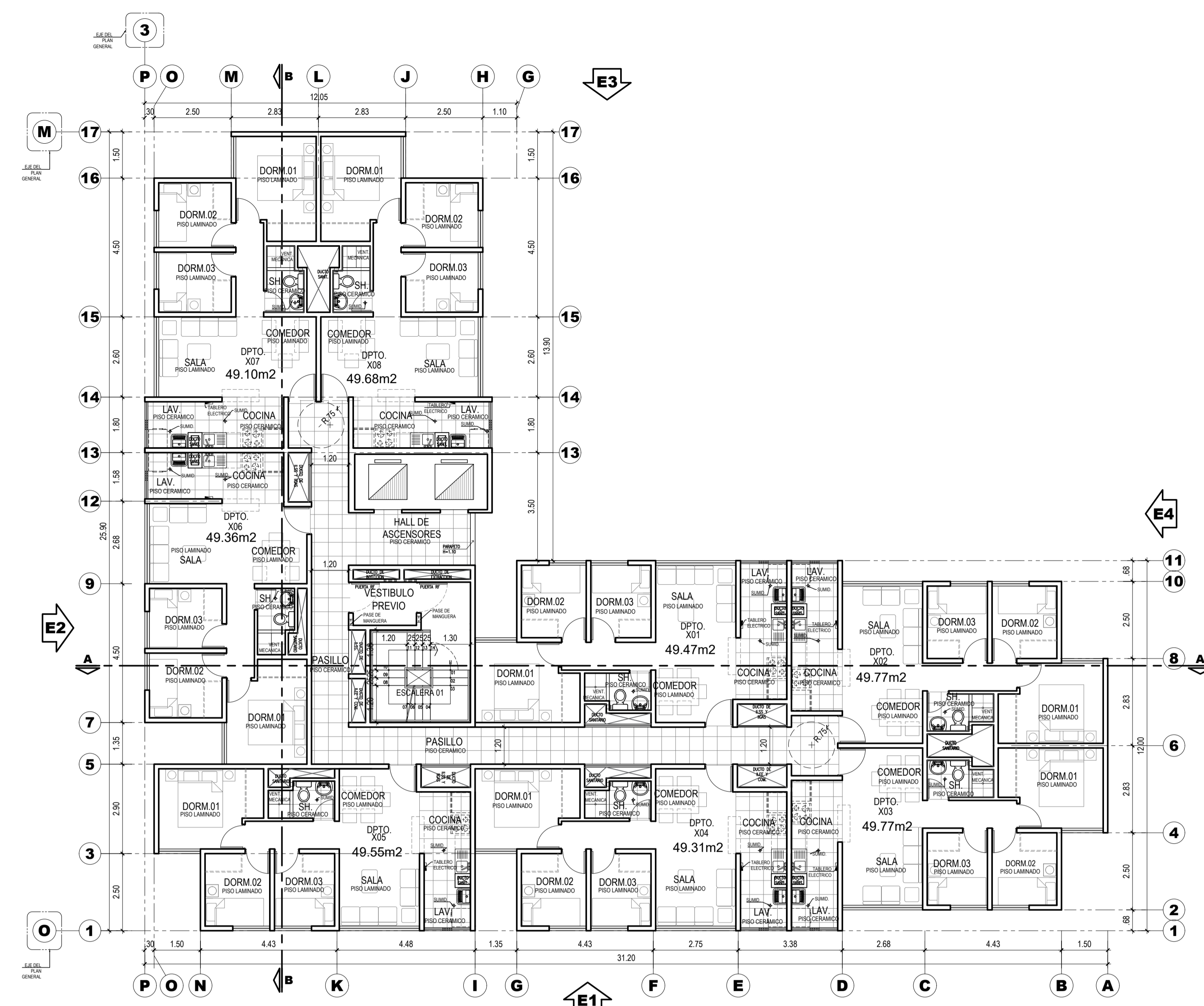
PLANTA TÍPICA PISOS 2 AL 21 ESCALA: 1/100
