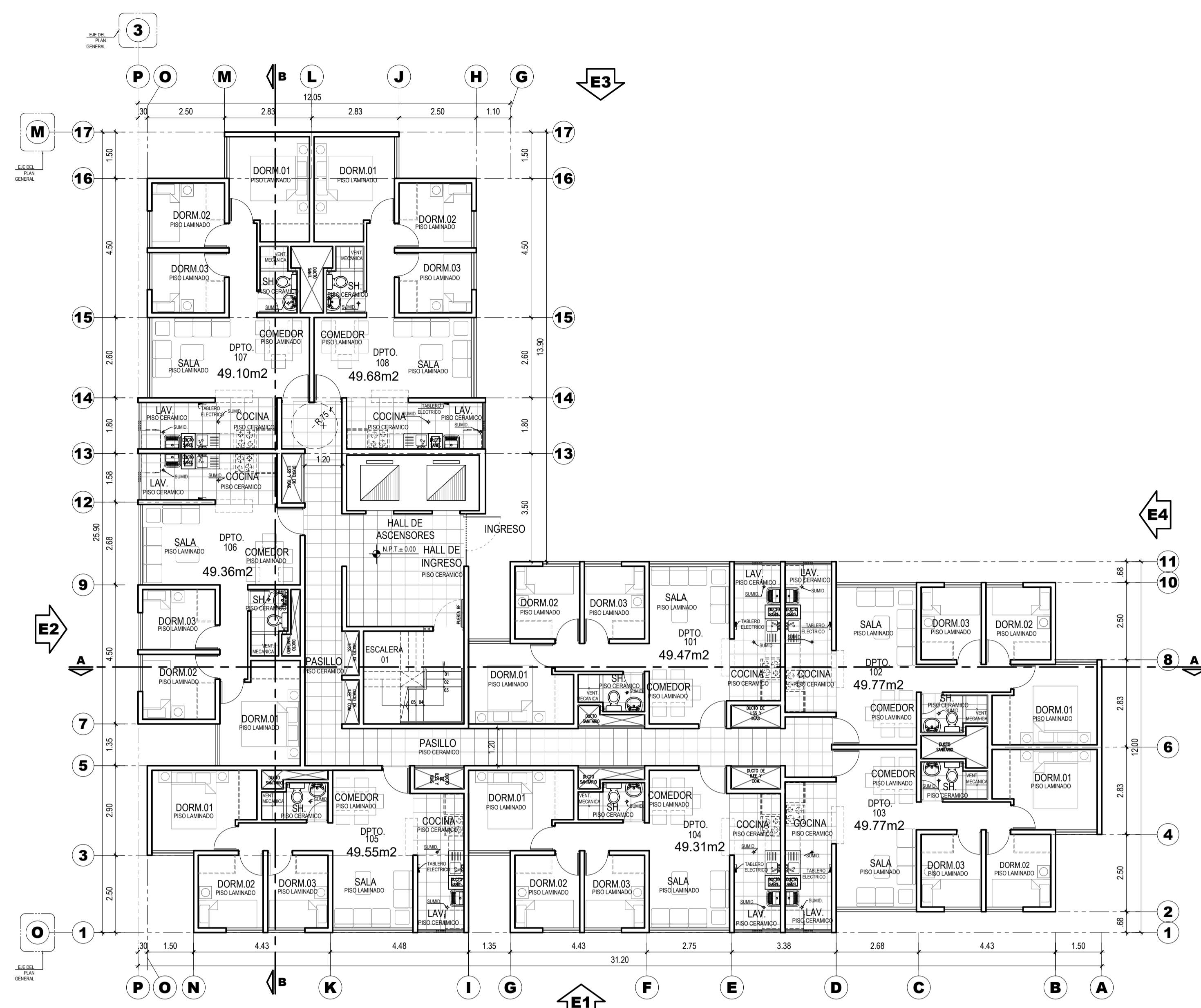
PLANTA PISO 1 ESCALA: 1/100
