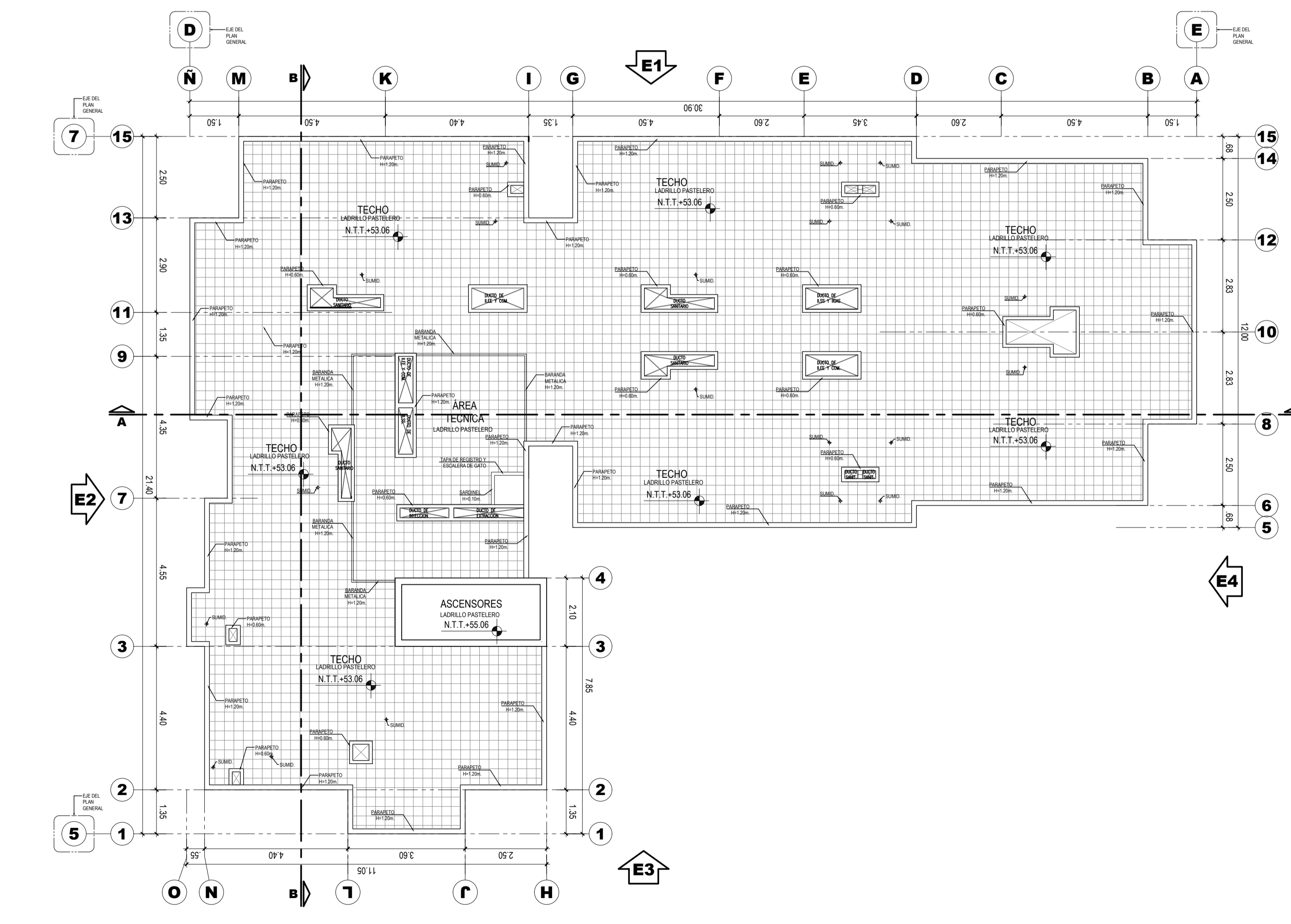
PLANTA TECHOS ESCALA: 1/100
