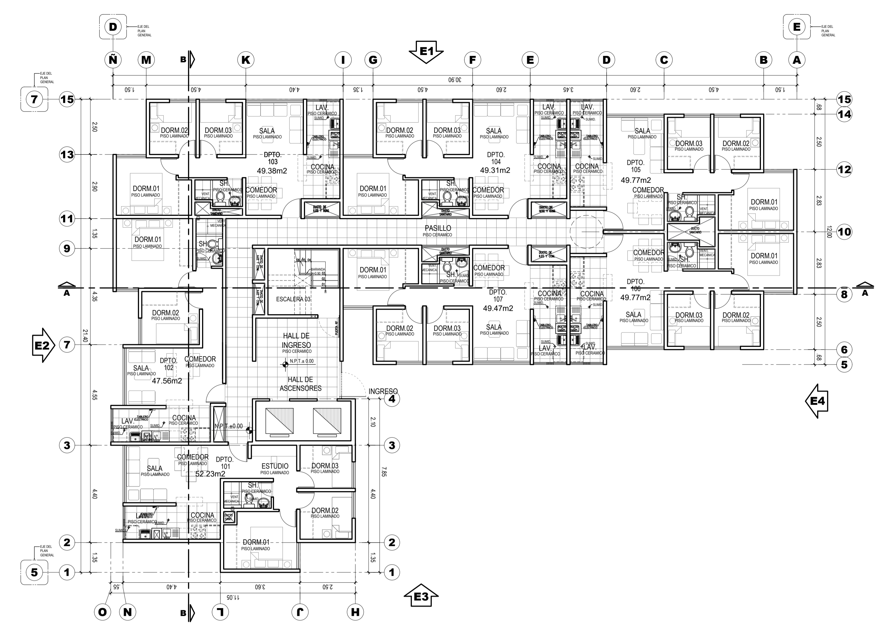
PLANTA PISO 1 ESCALA: 1/100
