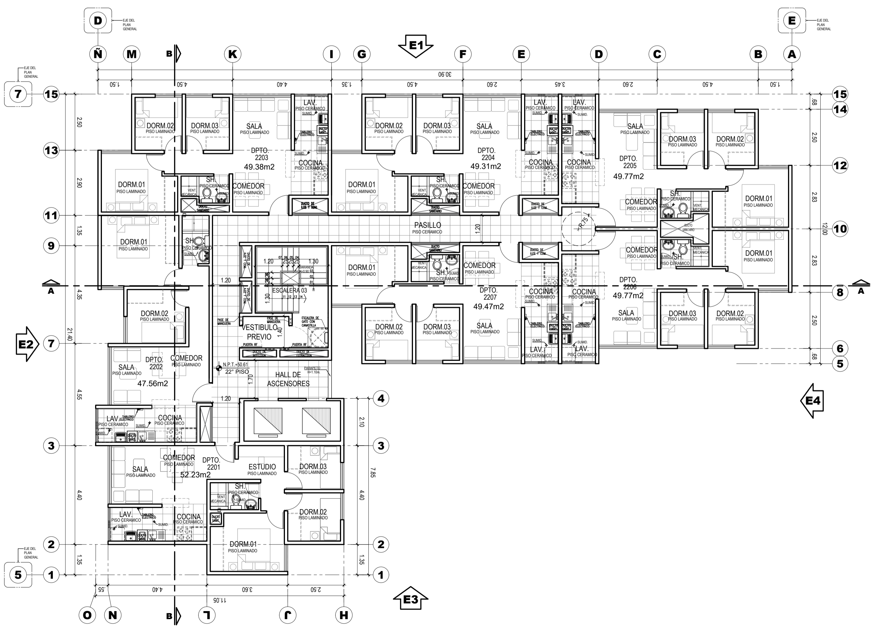
PLANTA TÍPICA DEL 22 ESCALA: 1/100
