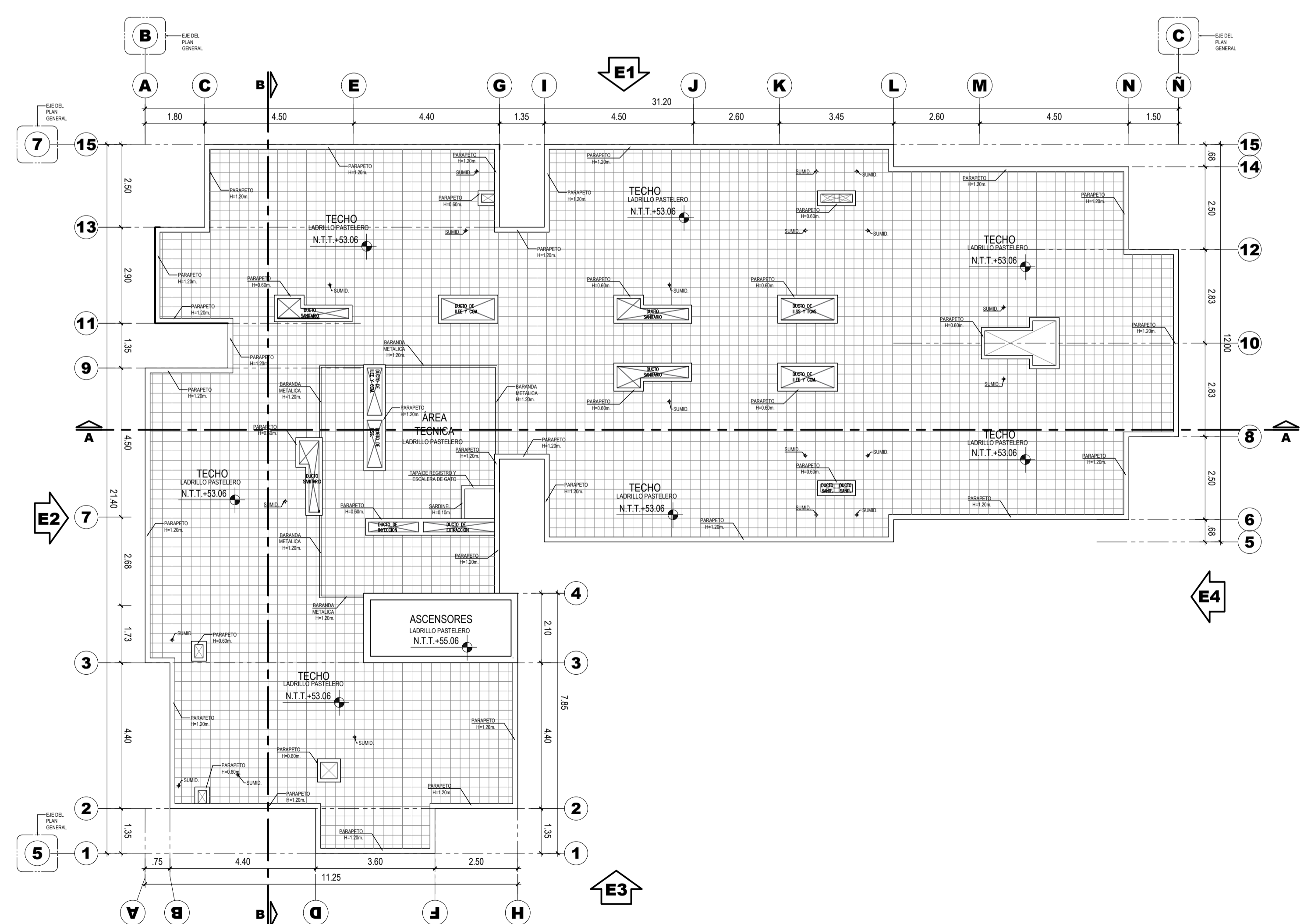
PLANTA TECHOS ESCALA: 1/100
