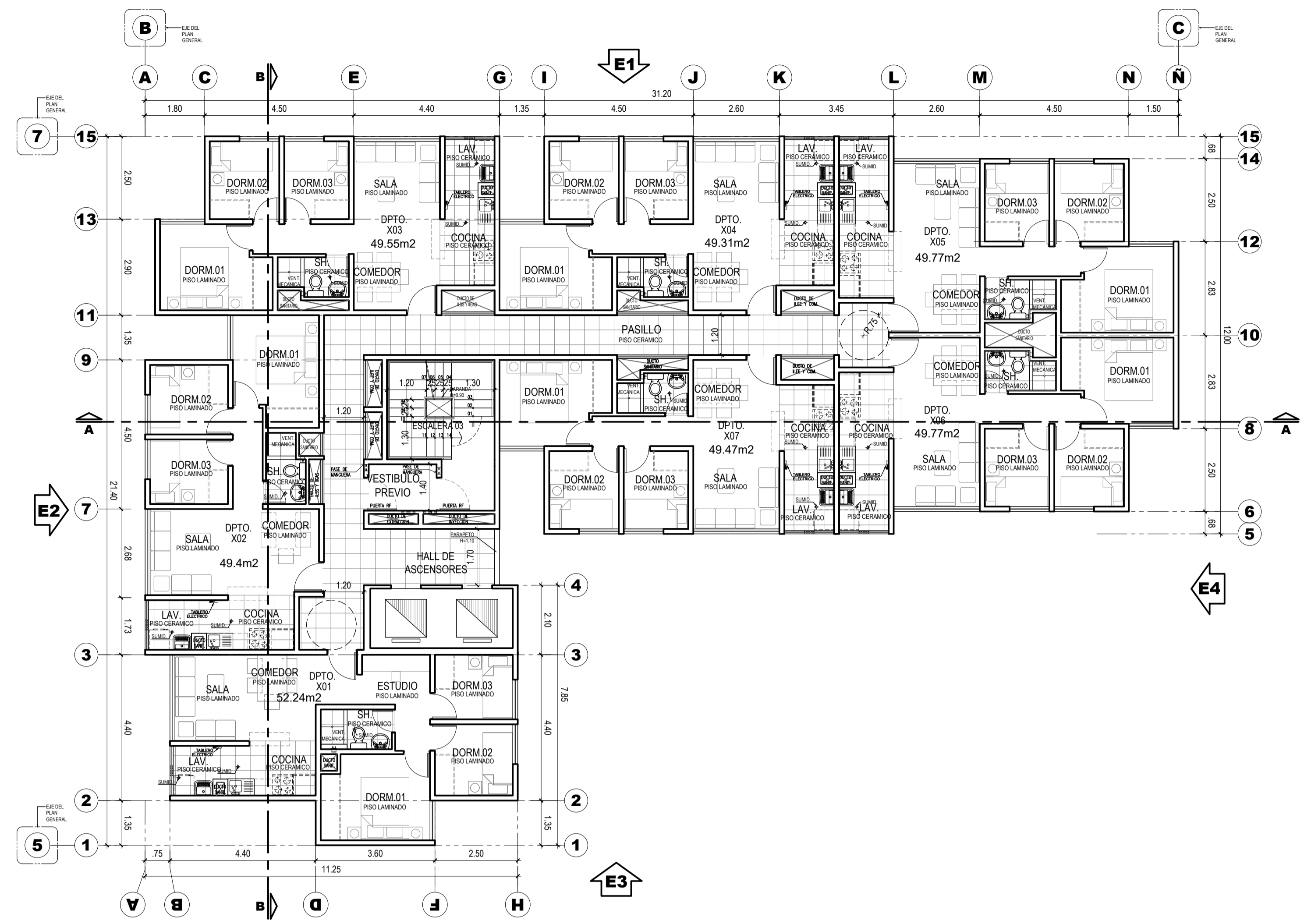
PLANTA TÍPICA DEL 2 AL 21 ESCALA: 1/100
