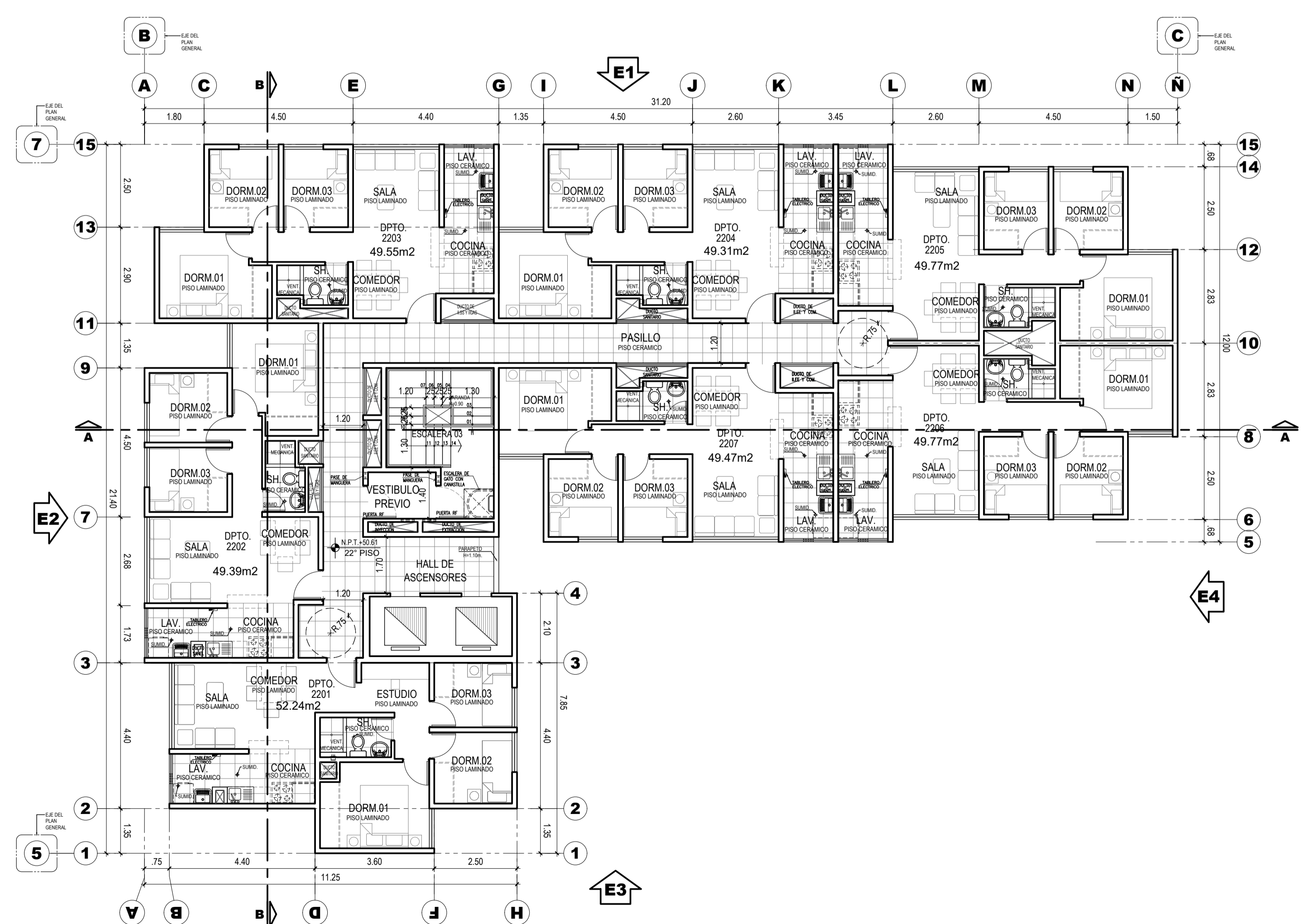
PLANTA TÍPICA DEL 22 ESCALA: 1/100
