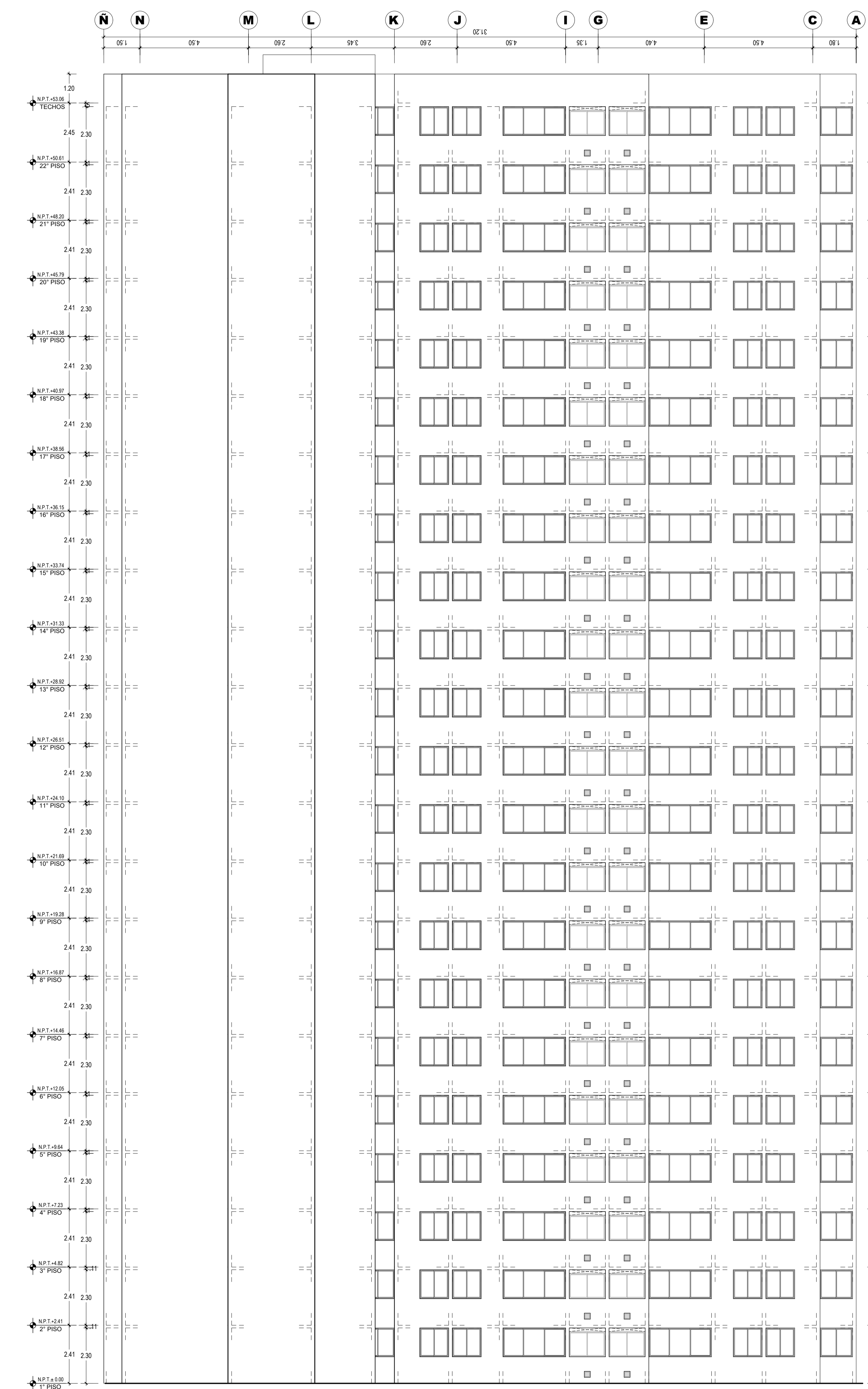
ELEVACION 3 ESCALA 1/100
