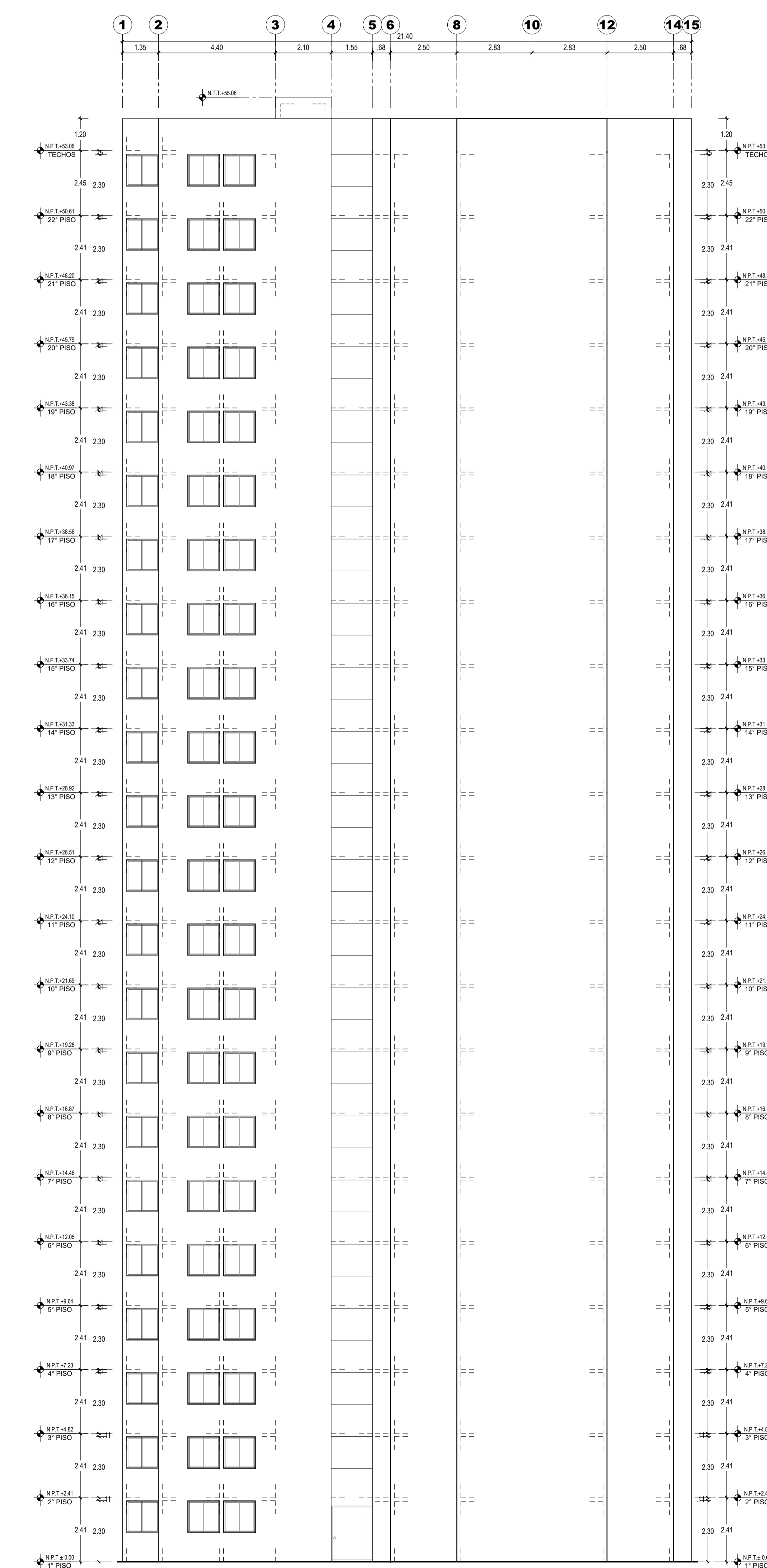
ELEVACION 4 ESCALA 1/100
